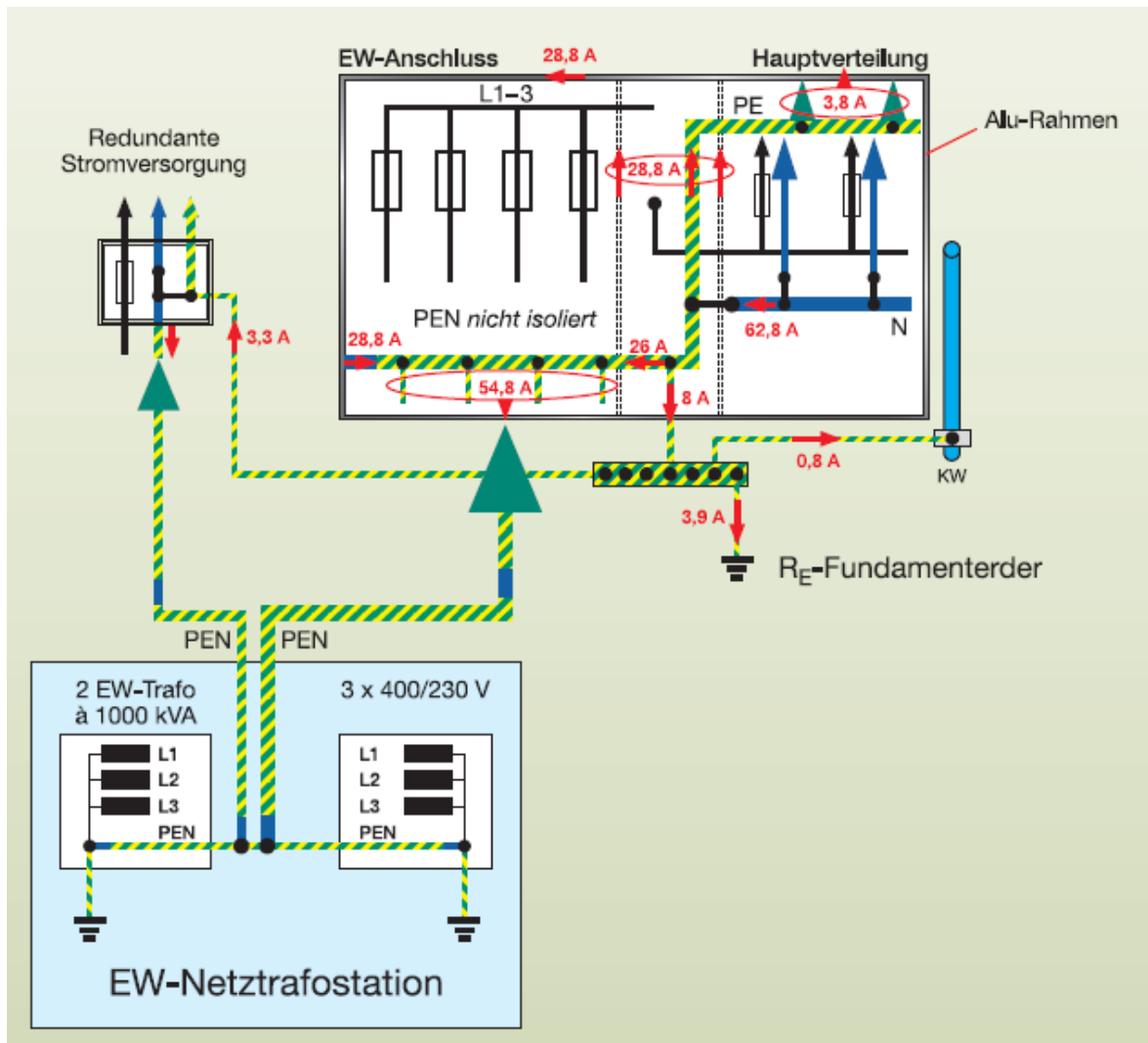
Bild 3. Gebäudestromversorgung und Stromversorgung für Sicherheitszwecke gemäss VKF-Brandschutzrichtlinie, Einspeisungen im TN-C-System. Magnetische Flussdichte 18 \mu\text{T} im Abstand von 20 cm um den Alu-Rahmen der Hauptverteilung.
