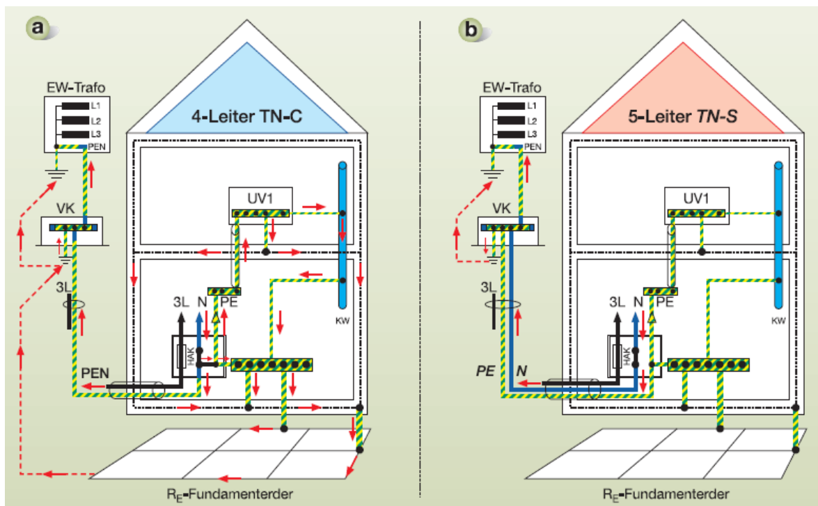
Bild 1. Vergleich TN-C versus TN-S
