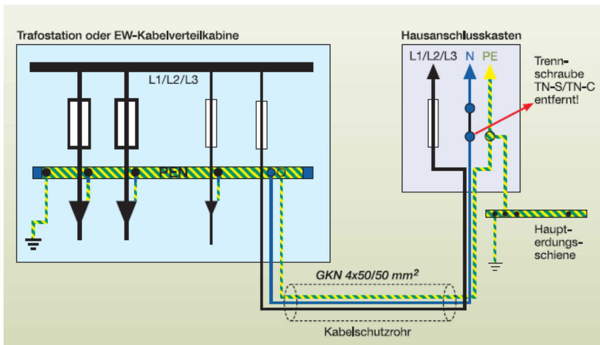
Bild 2. TN-S Anschluss von Fünfleiterkabeln an die bestehenden Betriebsmittel der Netzbetreiber. (Trafostation/Verteilkabine/KLV8)
