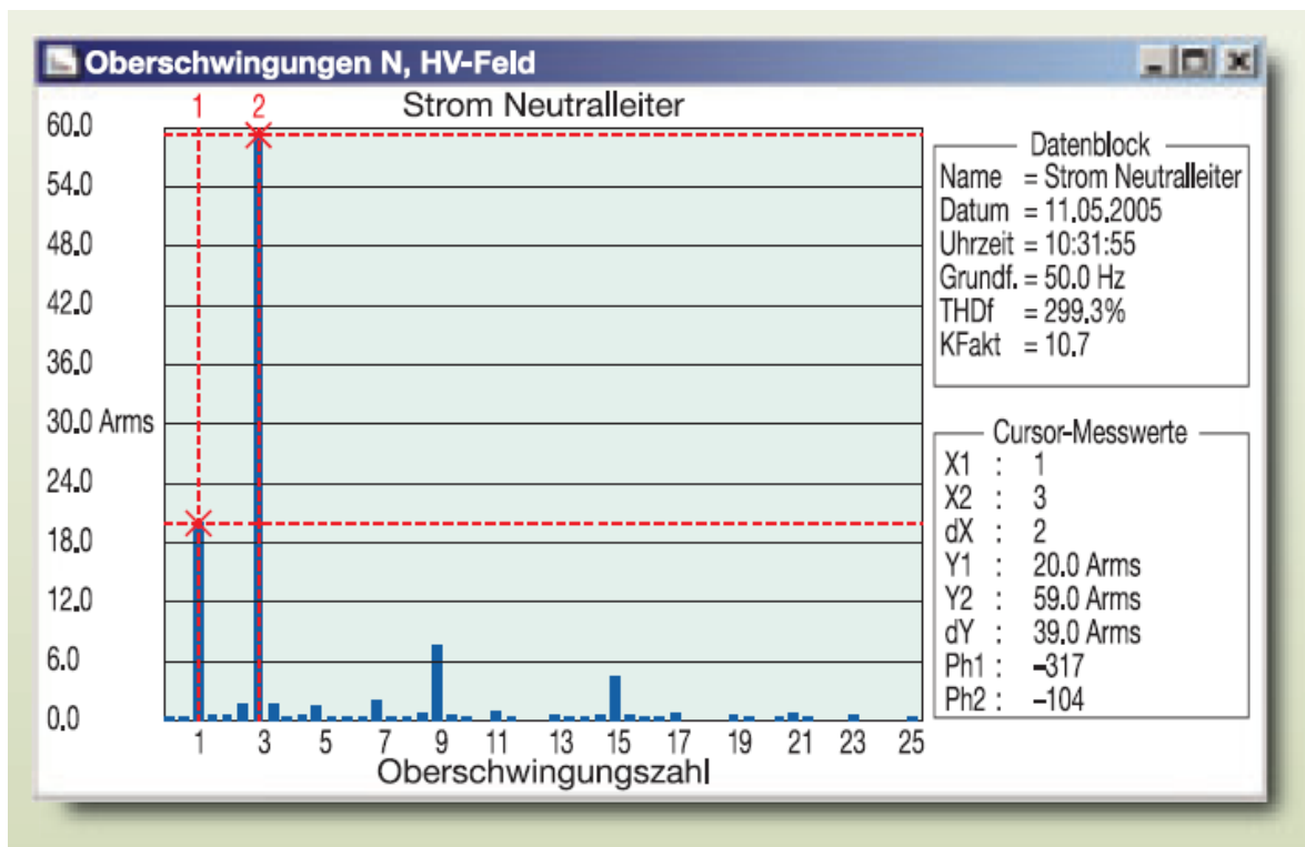
Bild 4 Die 3. Oberschwingung (150 Hz) dominiert mit 59 A den Strom im Neutralleiter. 50-Hz-Anteil: 20 A.
